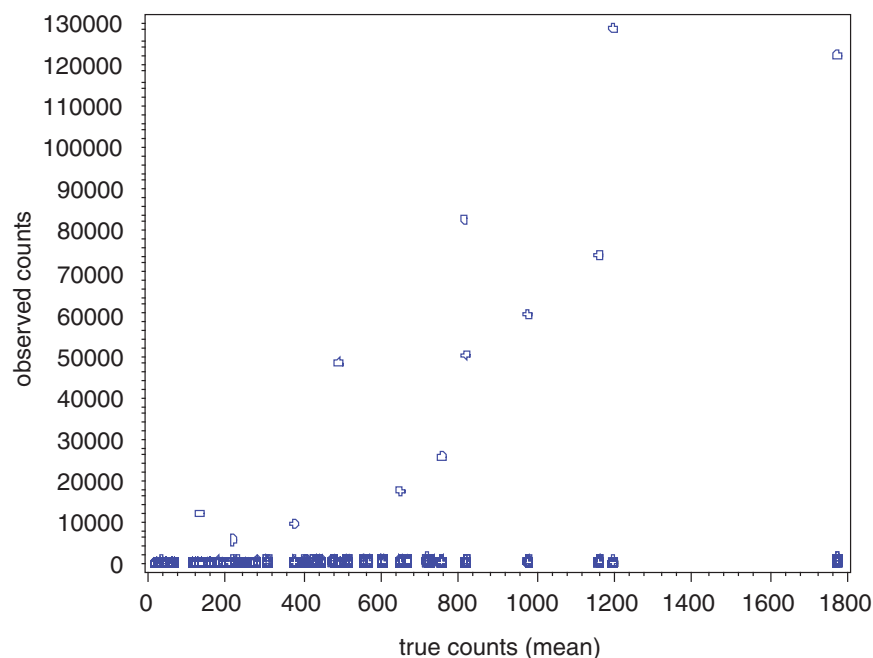
FIGURE B-6 Raw PCM data.
